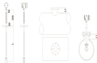
图（六）插入式外形图
