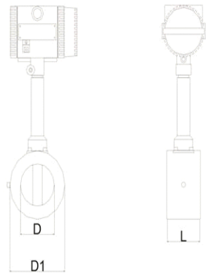
图 (二) 法兰卡装型外形图
