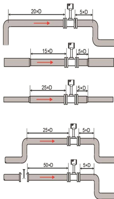
图（五）直管段示意图
