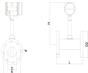
（表五）法兰连接型尺寸表
