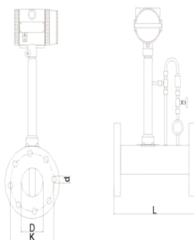
图(四) 温压补偿一体型外形图
